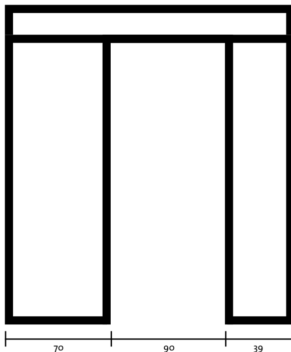
E12 METALON 200X220CM COM PORTA (INVERTIDO)
