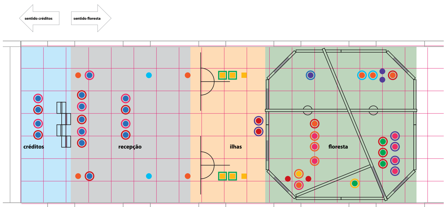
Mapa de iluminação - salão de exposições
